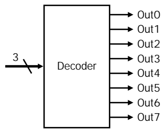
a. A 3-bit decoder
